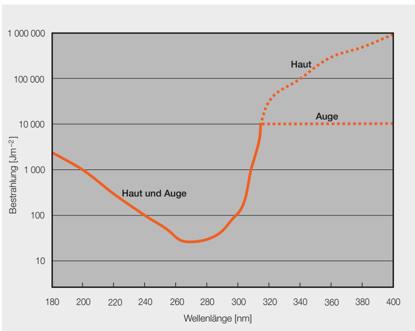
Figur 1 UV-Strahlungs-Grenzwerte innerhalb von 8 Stunden (Arbeitstag). Grafische Darstellung der Bestrahlungsgrenzwerte aus Tabelle 2 (Seite 148).
