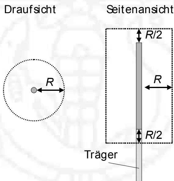
Bild 1b: Sicherheitsabstände für Rundstrahlantennen
