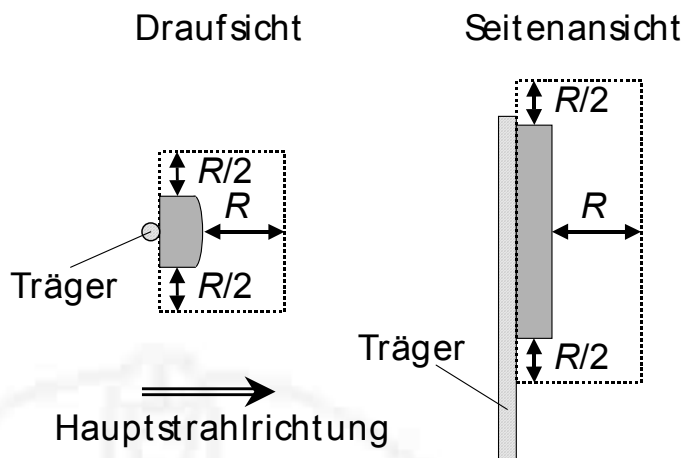
Bild 1a: Sicherheitsabstände für Richtantennen
