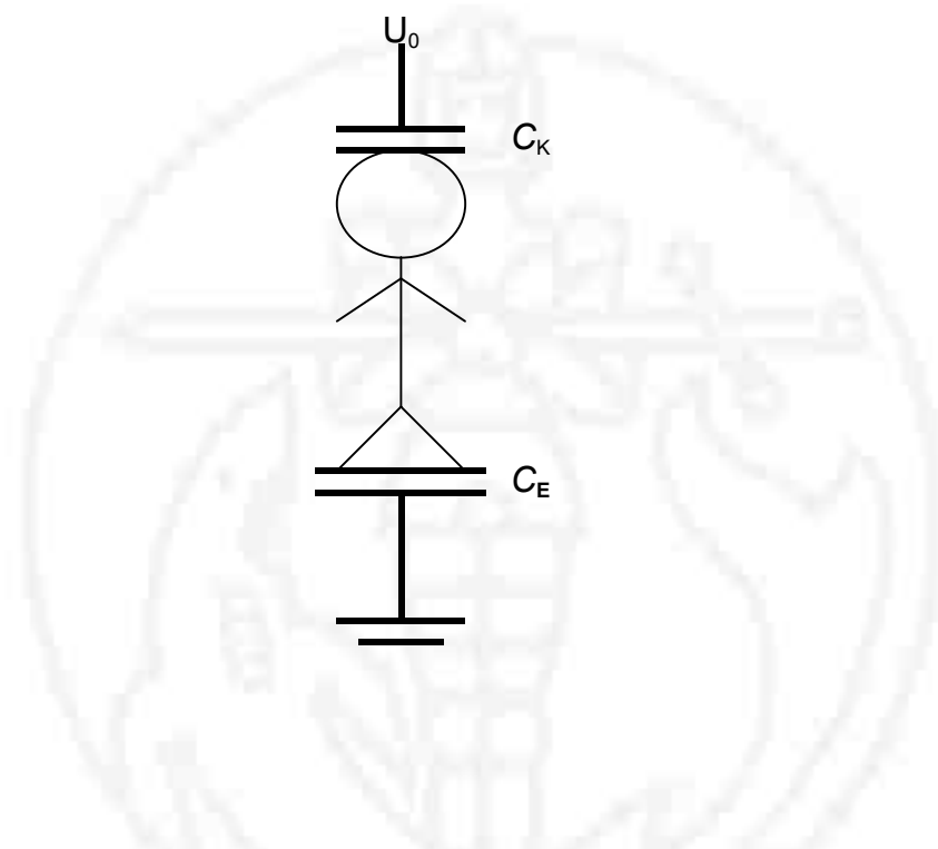
Abbildung 1: Ersatzschaltbild kapazitive Kopplung
